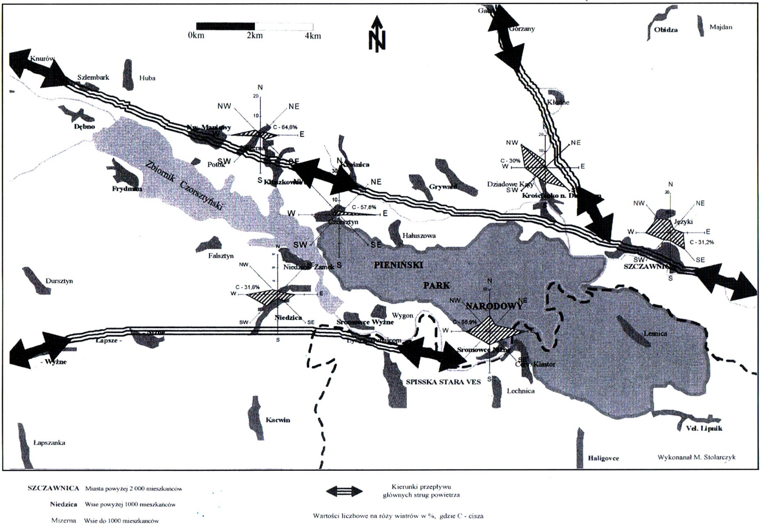
Rys.4. CZĘSTOTLIWOŚĆ KIERUNKÓW WIATRÓW W % ORAZ GŁÓWNE KANAŁY UPRIWILEJOWANYCH STRUG POWIETRZA
