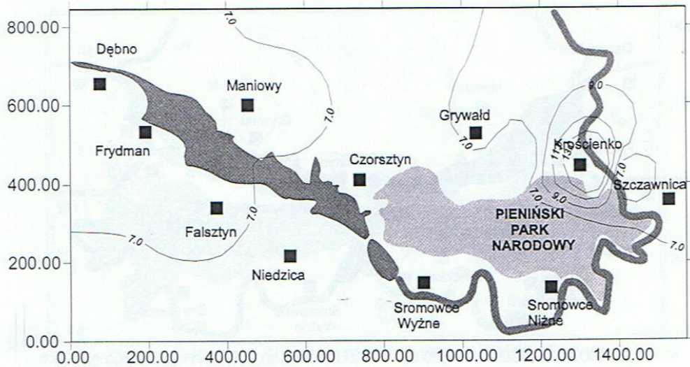
Ryc. 7. Rozkład przestrzenny dwutlenku azotu w lipcu 1996 r. Spatial distribution of \text{NO}_2 in July 1996.
