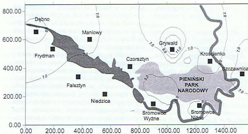
Ryc. 9. Rozkład przestrzenny dwutlenku azotu w lutym 1996 r. Spatial distribution of \text{NO}_2 in february 1996.
