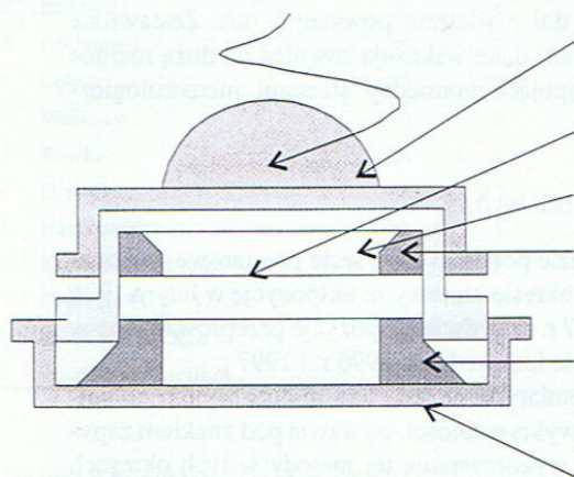
Ryc. 2. Przekrój poprzeczny próbnika. Cross-section of a sampler.
