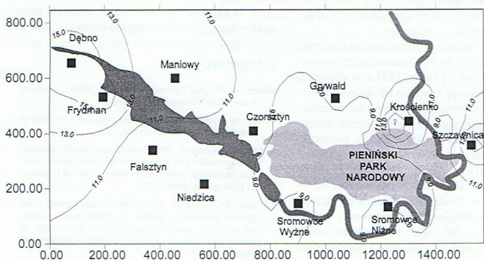
Ryc. 10. Rozkład przestrzenny dwutlenku azotu w lutym 1997 r. Spatial distribution of \text{NO}_2 in february 1997.
